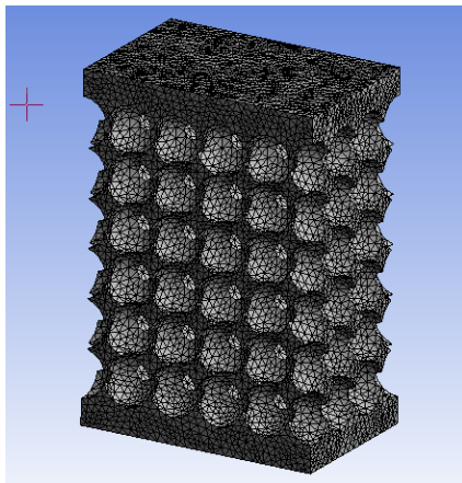
Fig. 10 Mesh
